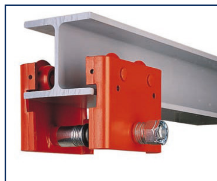
Carro traslación manual
